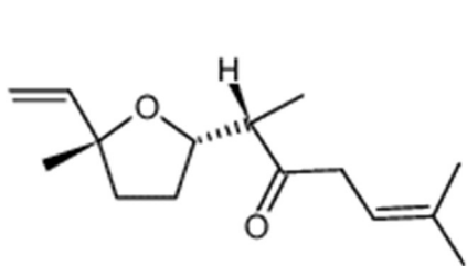
davanone
