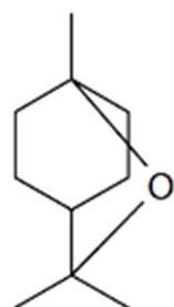
1,8 cineol
