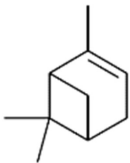
\alpha -pinen
