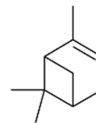
\alpha -pinen, 63-83 %
