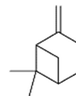
\beta -pinen
