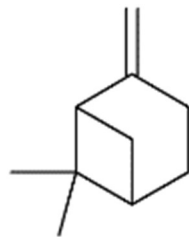
\beta -pinen
